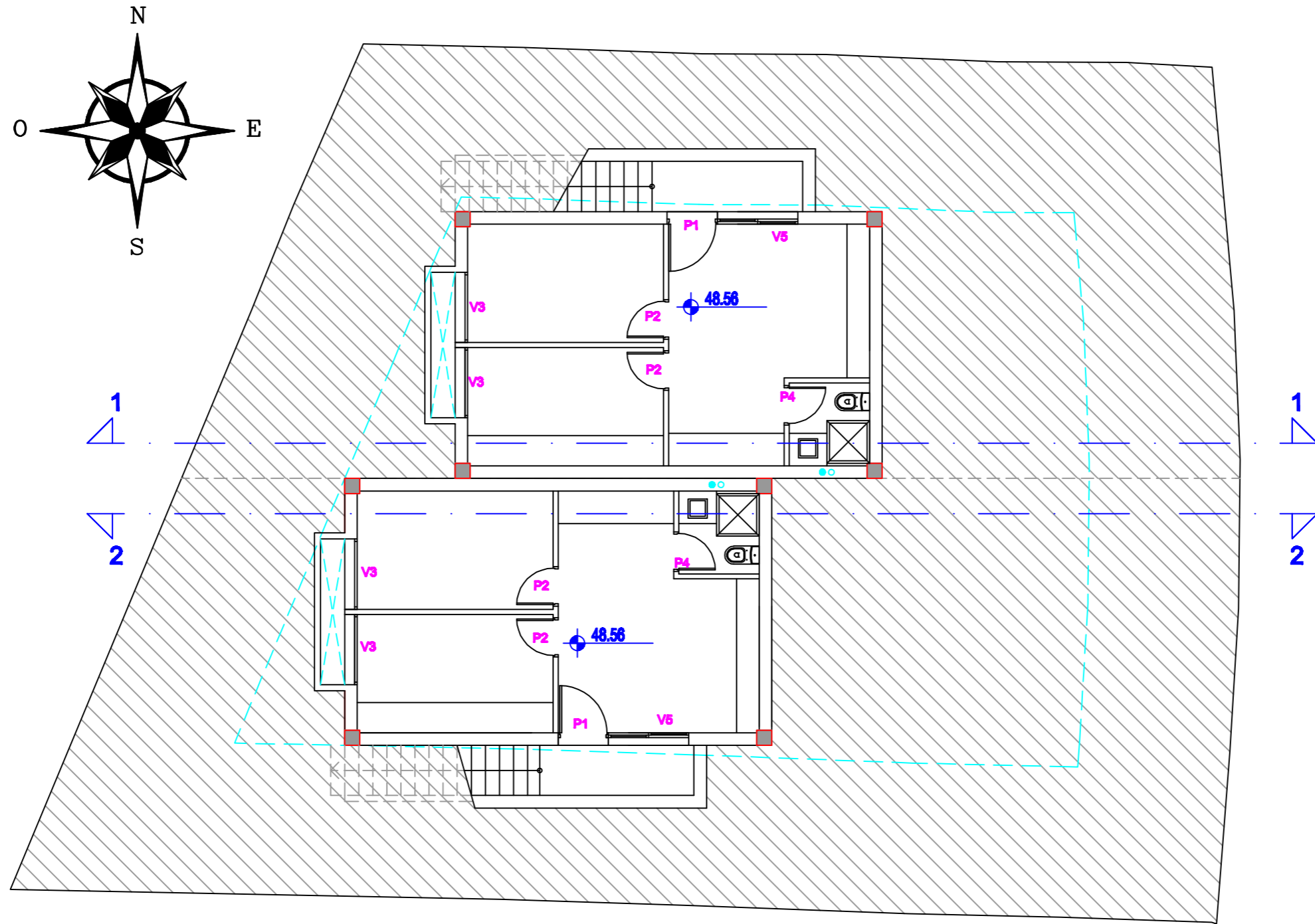
PLANTA SOTANO
