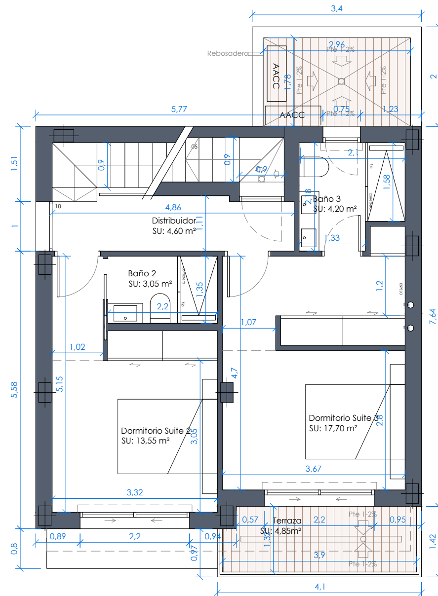
PLANTA PRIMERA
