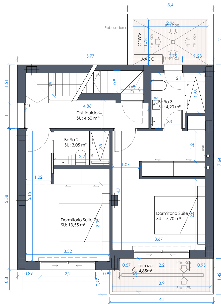
PLANTA PRIMERA
