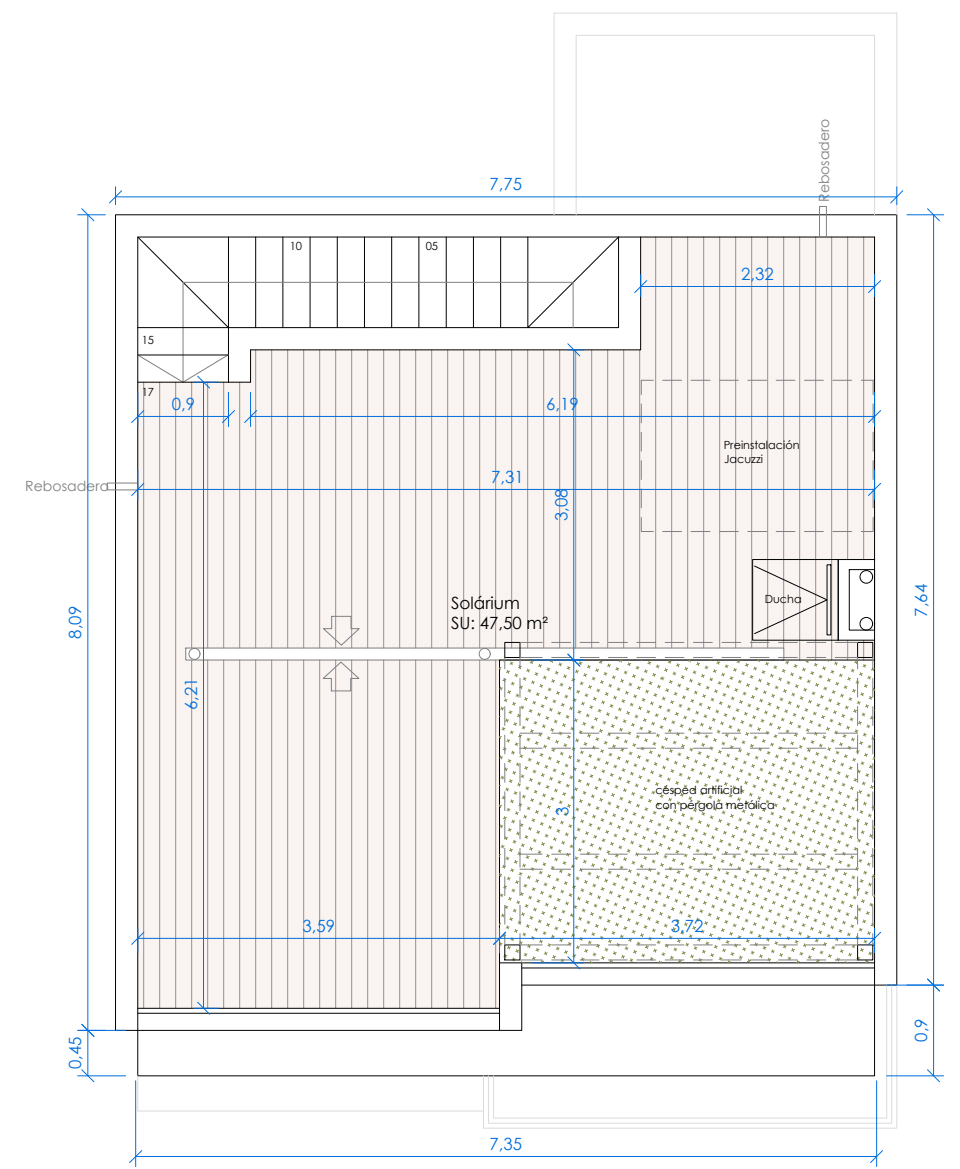
PLANTA CUBIERTA
