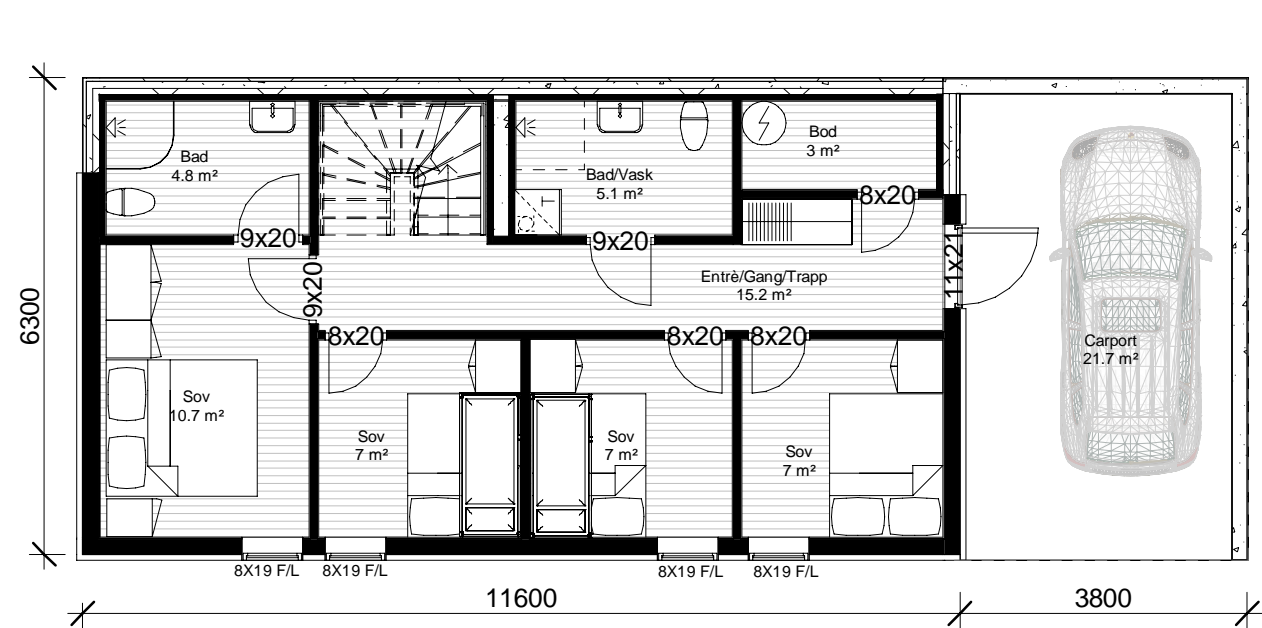
Et. 1 1 : 100
