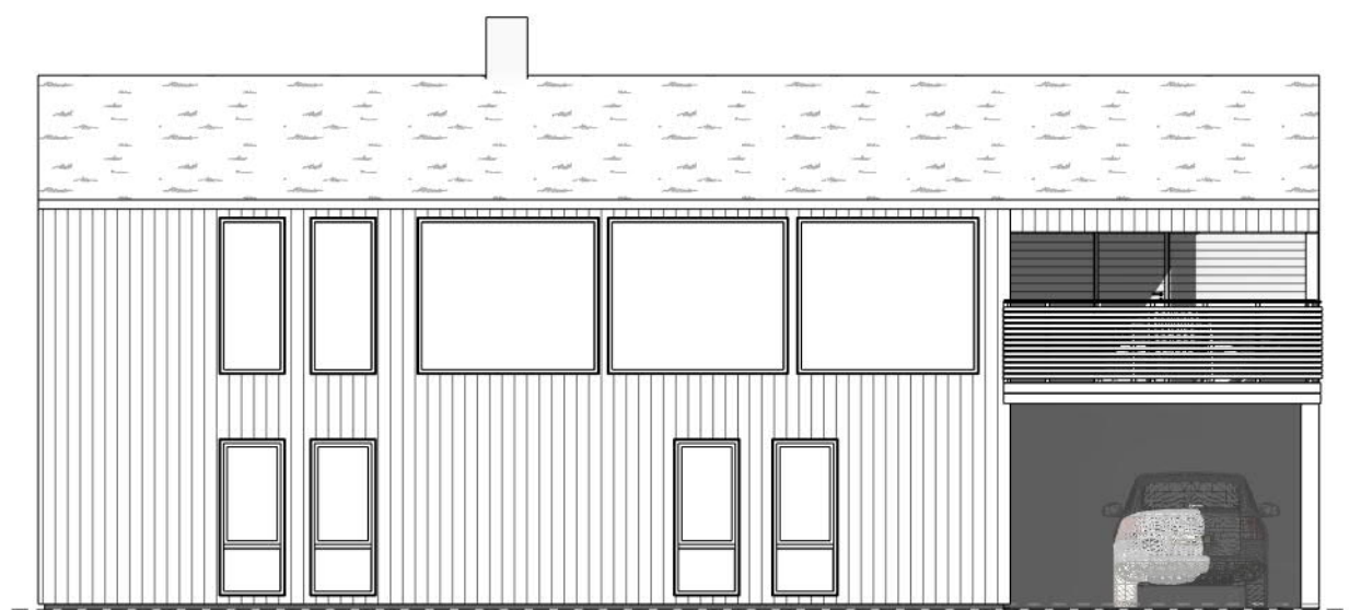
Nord 1 : 100
