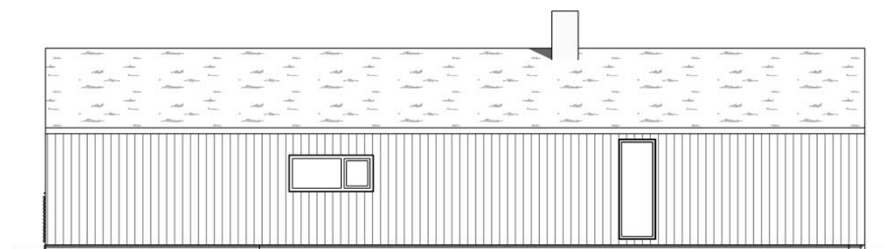
Sør 1 : 100
