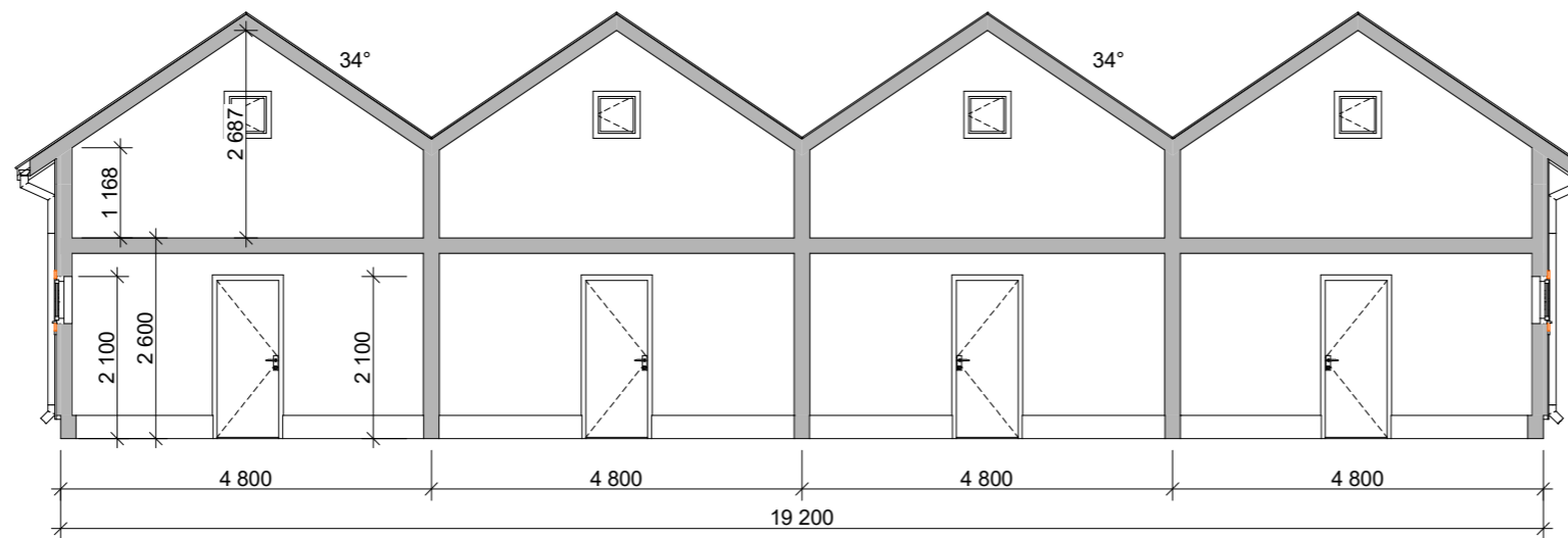
Snitt A-A
