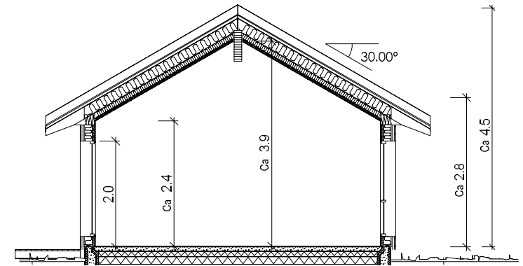
SNITT B - B
