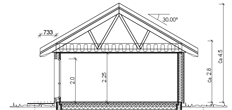
SNITT C - C
