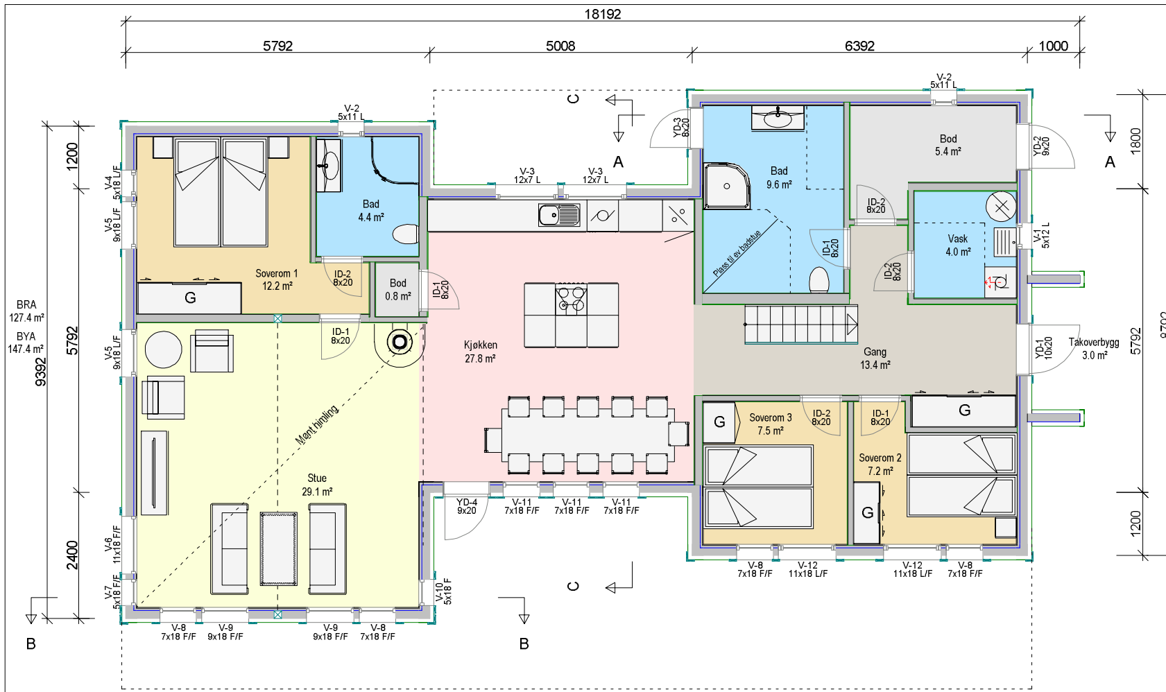
PLAN 1 ETASJE
