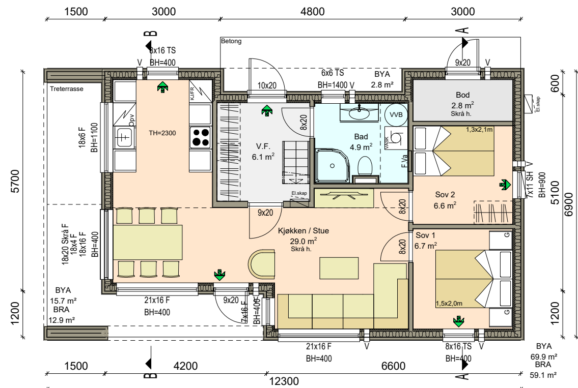
Plan 1 etg.
