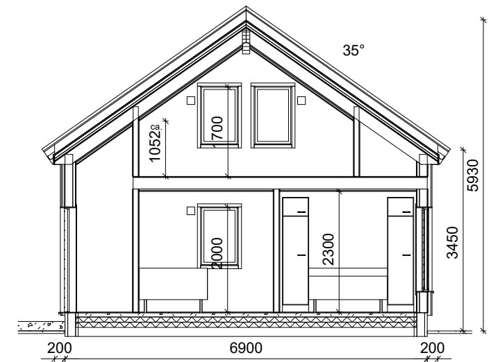
Snitt A-A
