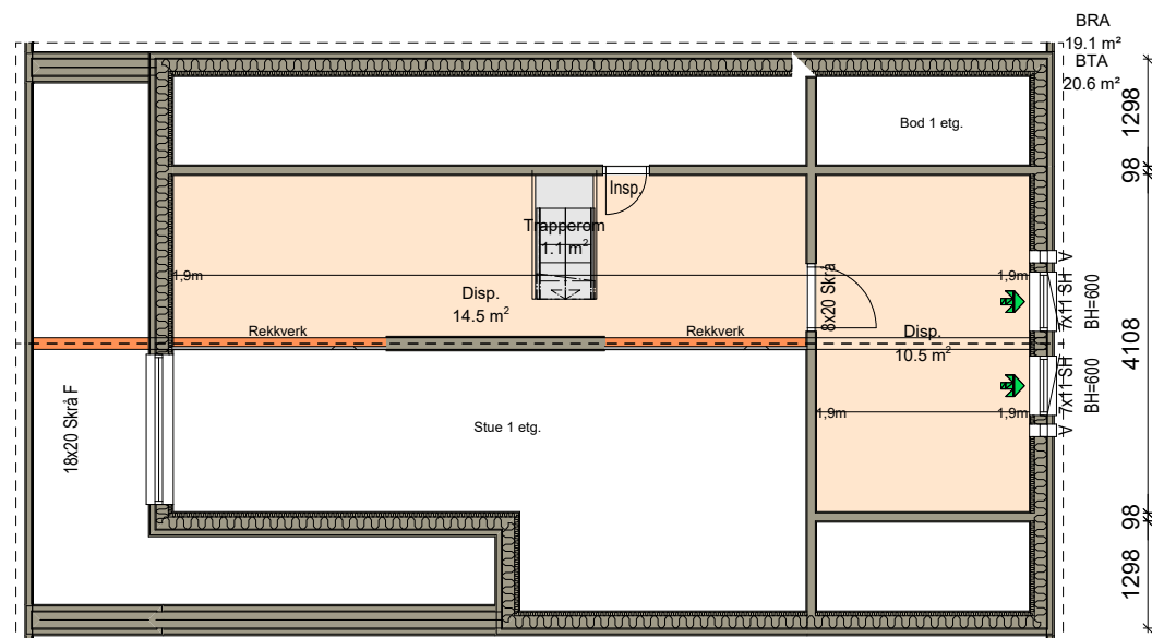
Plan loft
