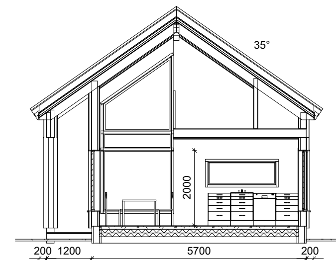
Snitt B-B
