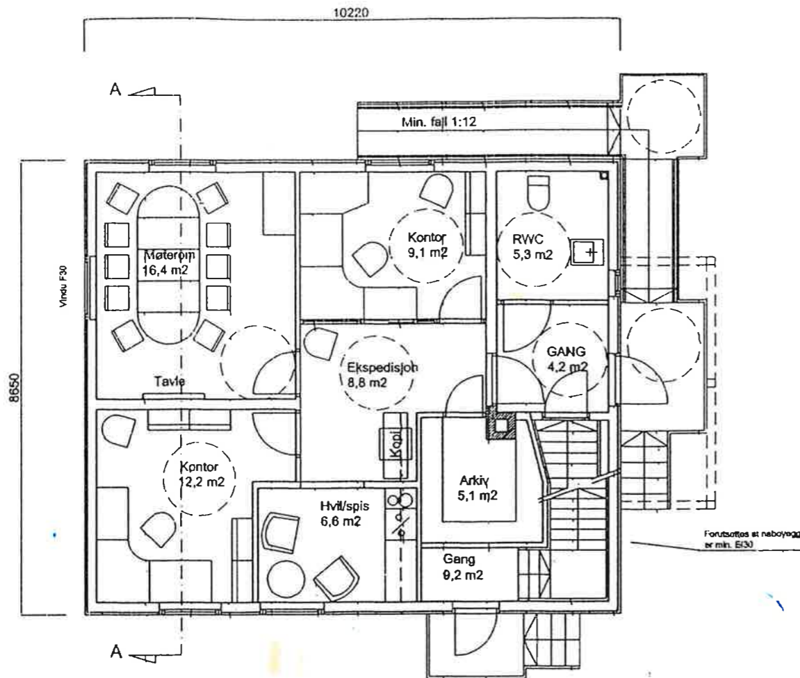
PLAN 1.ETG.
