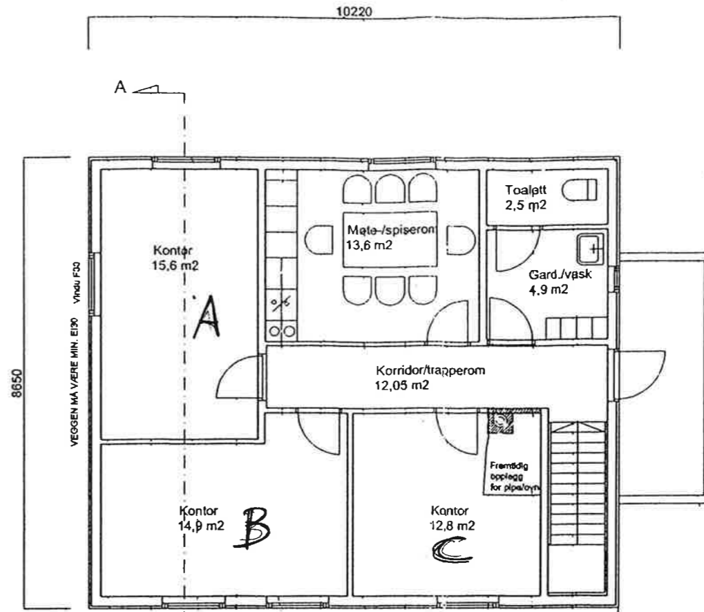
PLAN 2.ETG.
