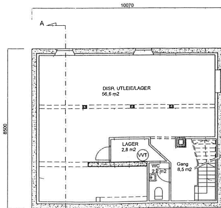
PLAN U.ETG.
