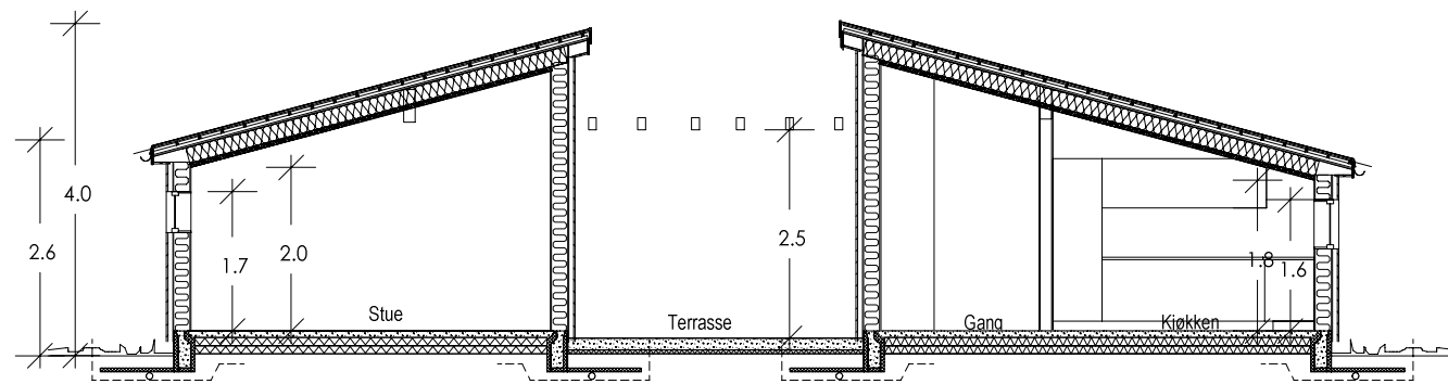
Snitt A-A
