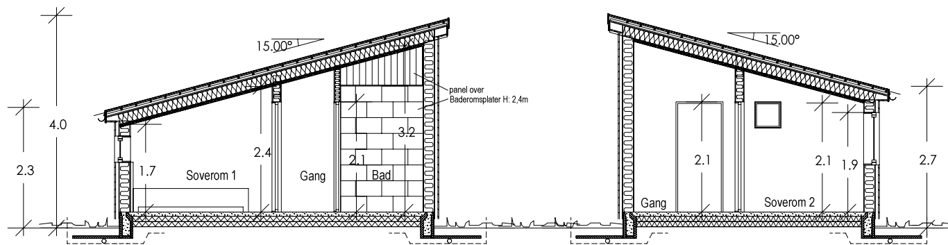
Snitt B-B
