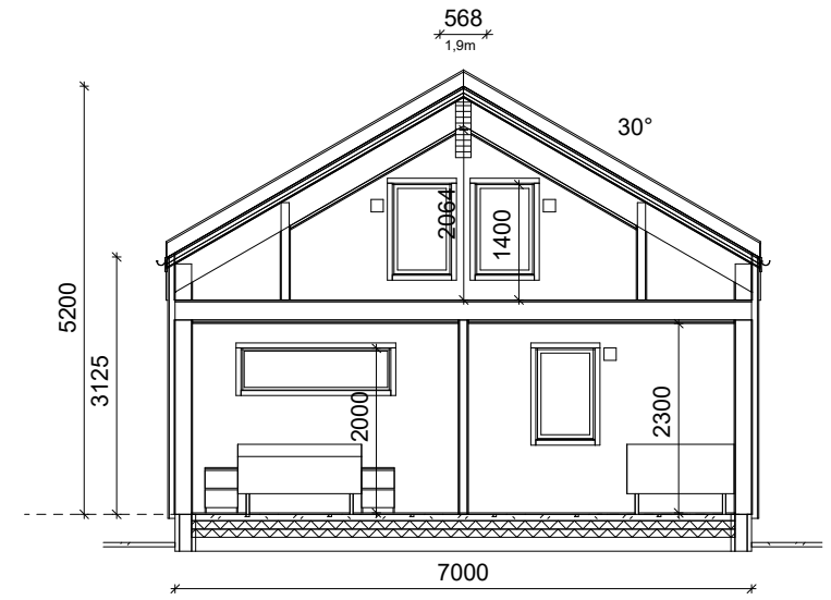
SNITT A-A
