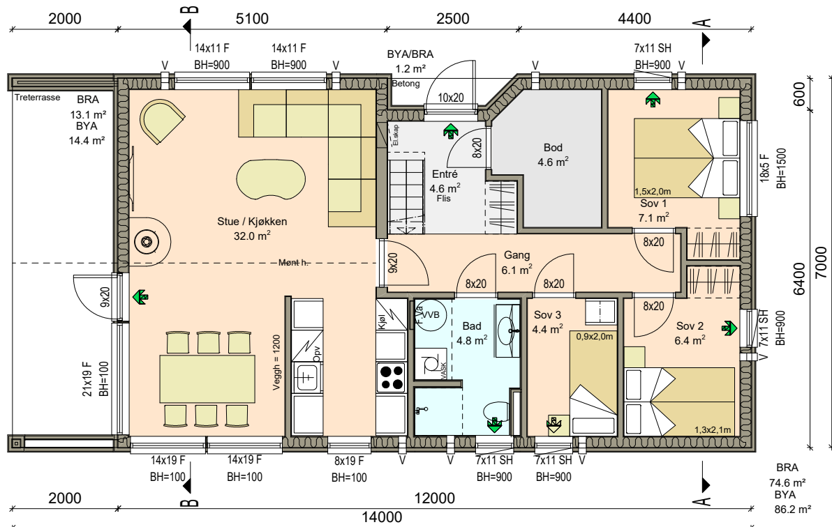
Plan 1 etg.
