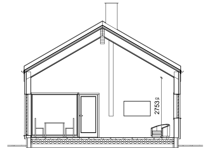
SNITT B-B
