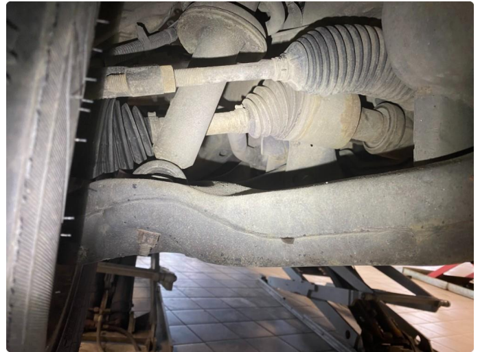
3.1 Hjullager høyre foran skiftet
