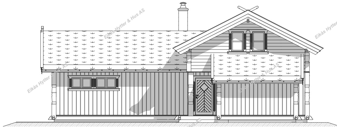
Fasade 4
