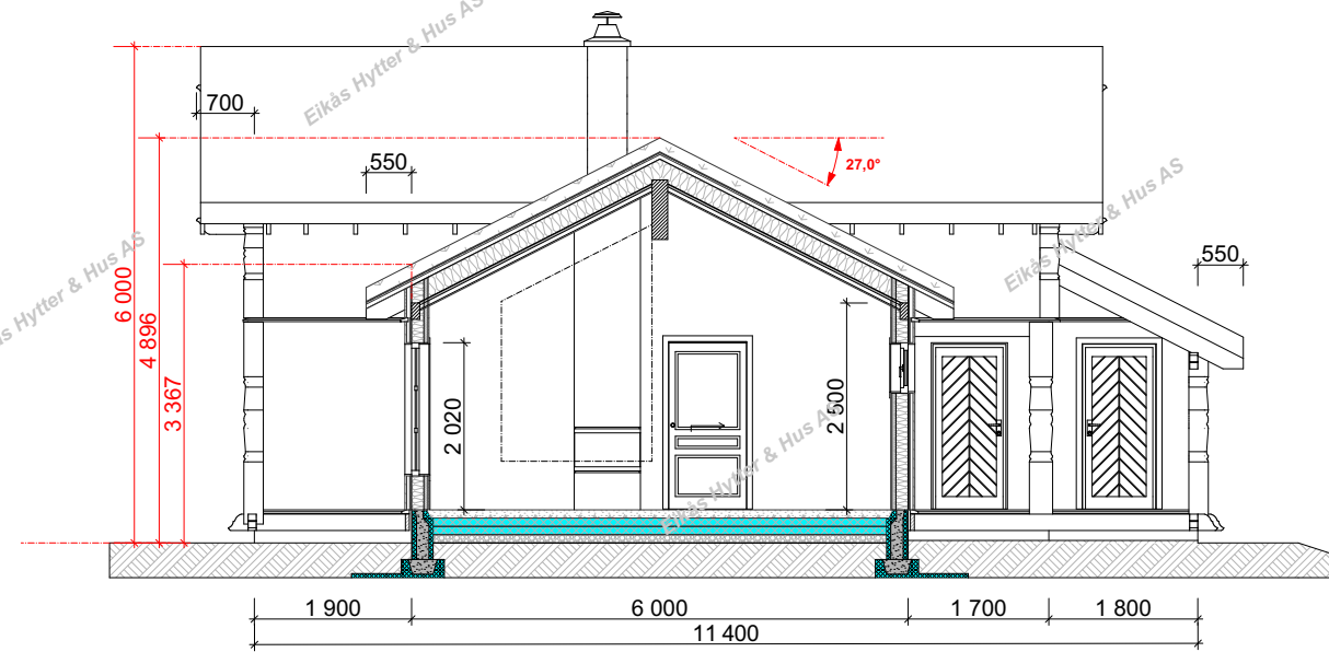
Snitt A-A
