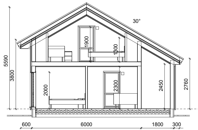
Snitt A-A
