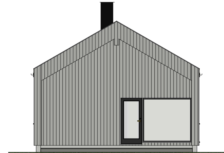
Fasade mot vest
