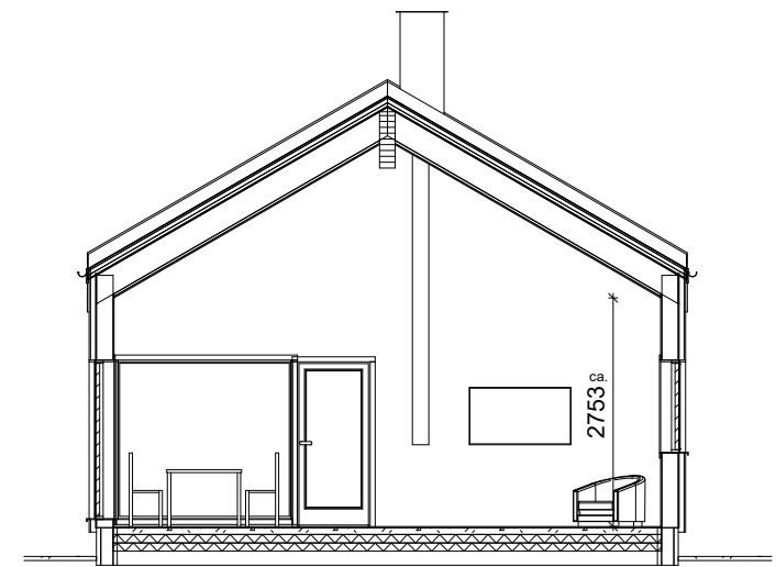
SNITT B-B
