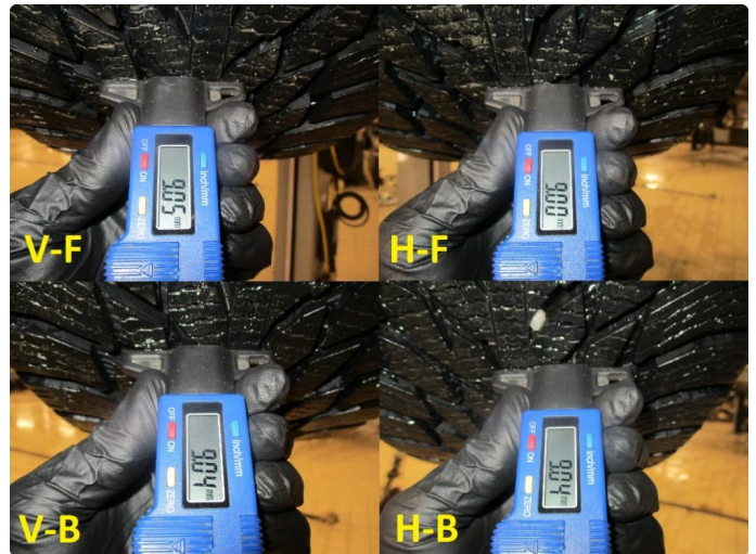
1.2 Mønsterdybde målt på vinterdekk 09.03.2023 ved 2946km
