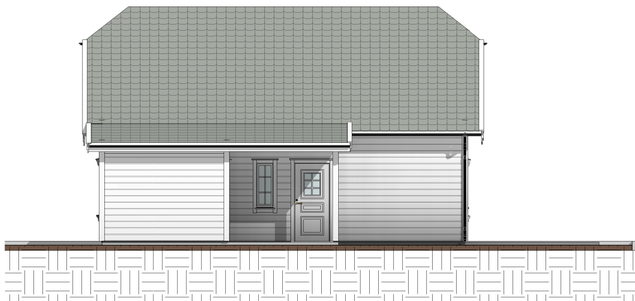
Fasade mot nord 1 : 100
