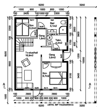
HOVEDPLAN
