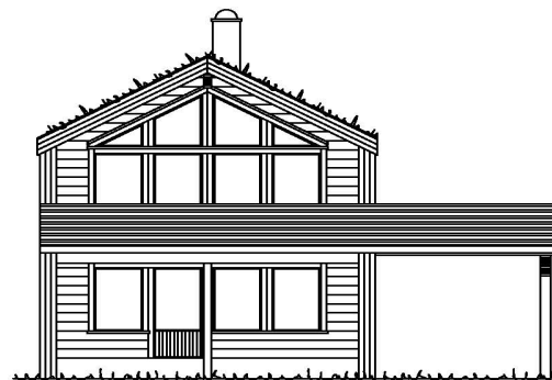
FASADE MOT
