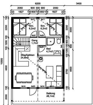
LOFTSPLAN
