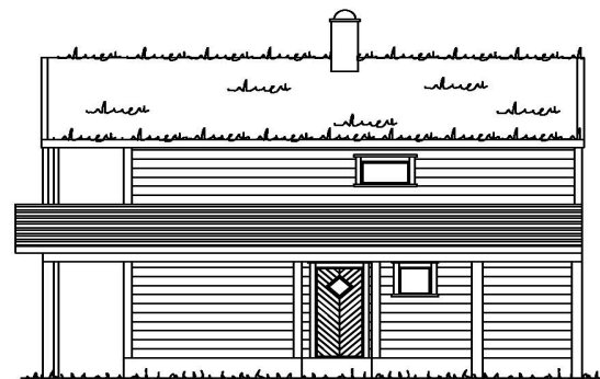
FASADE MOT
