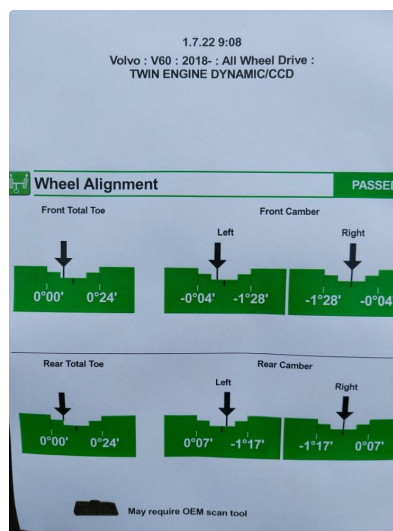
2.1 4-hjulsmåling/forstillingskontroll
