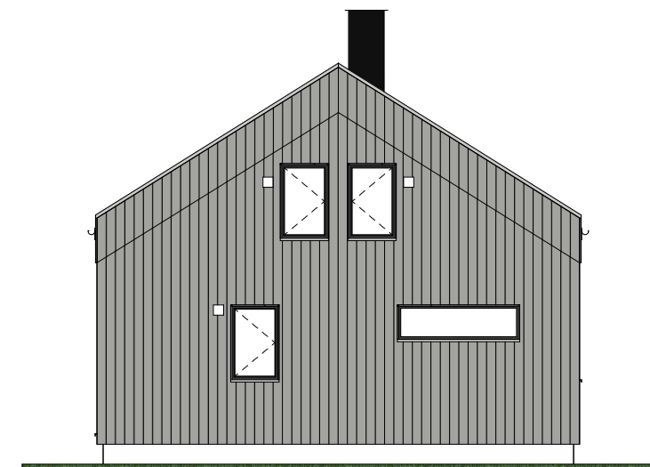
Fasade mot sør-øst
