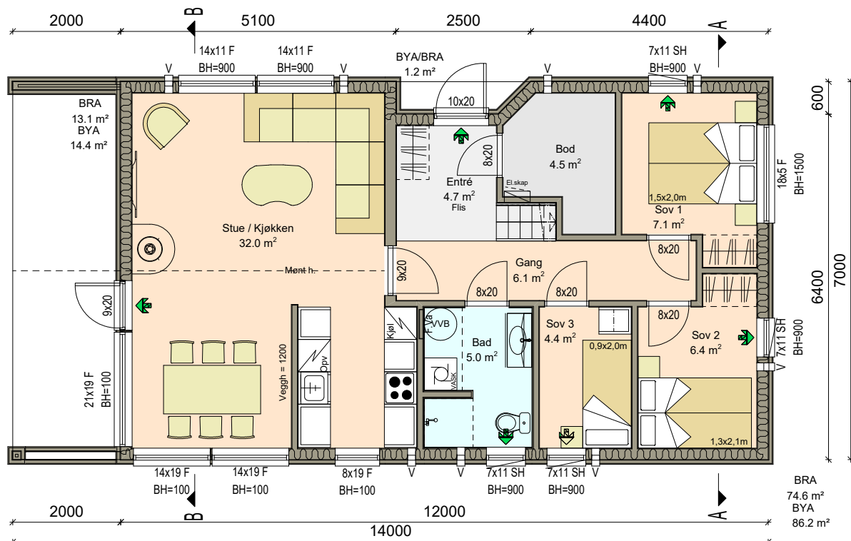
Plan 1 etg.
