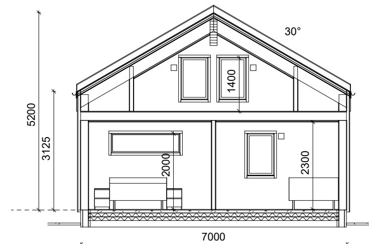
SNITT A-A
