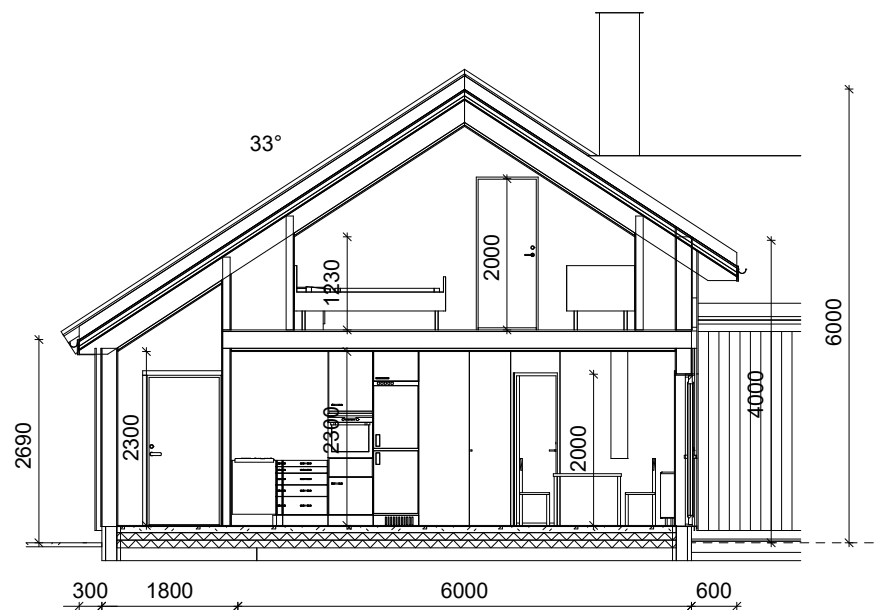
Snitt A-A
