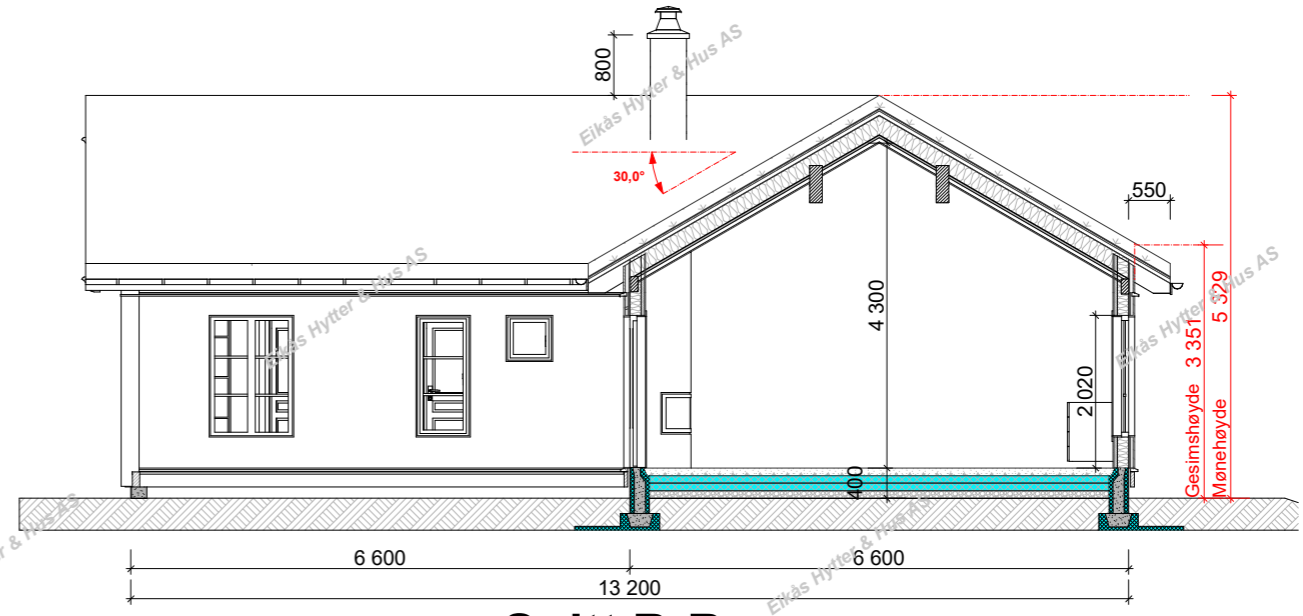
Snitt B-B
