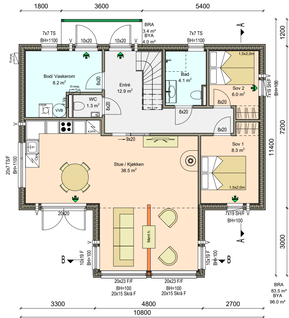
Plan 1 etg.
