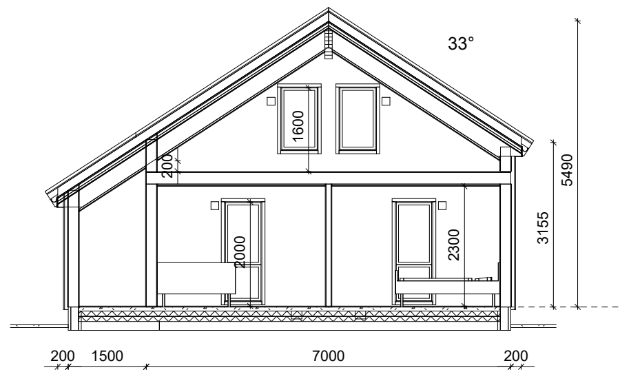
Snitt C-C
