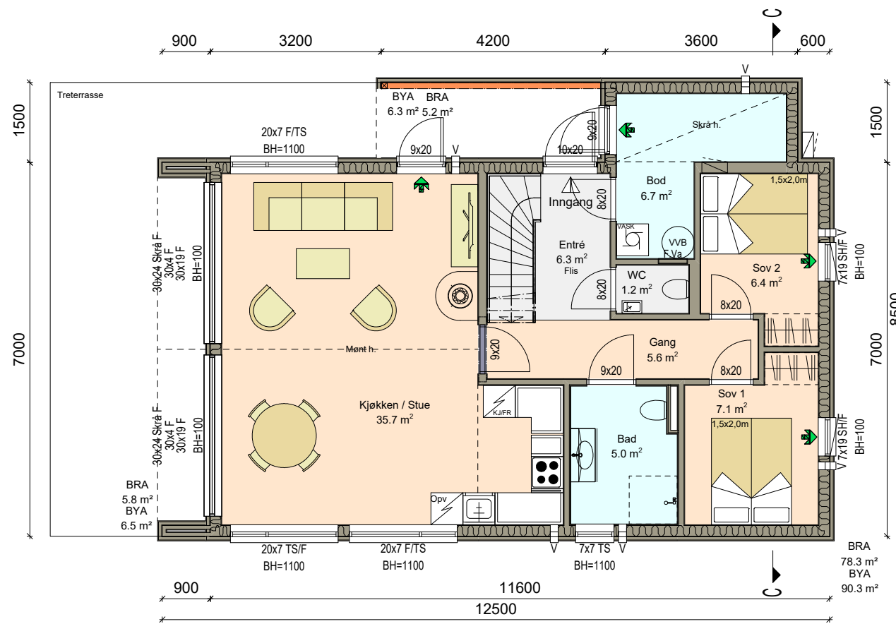
Plan 1 etg.
