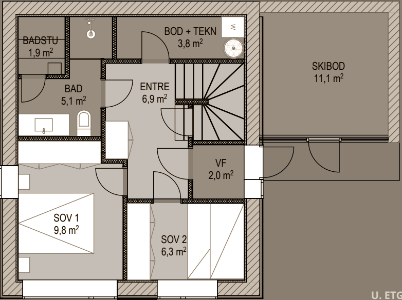
U. ETG
