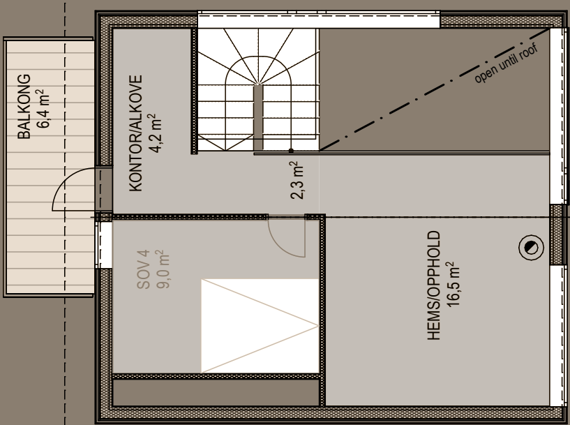
LOFT
