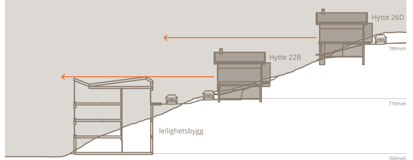
Snitt CC
