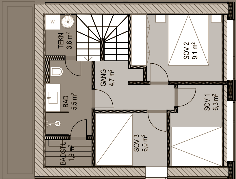
U. ETG
