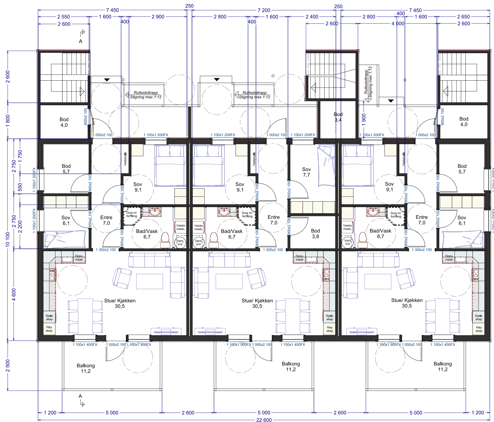
PLANTEGNING 1. ETASJE
