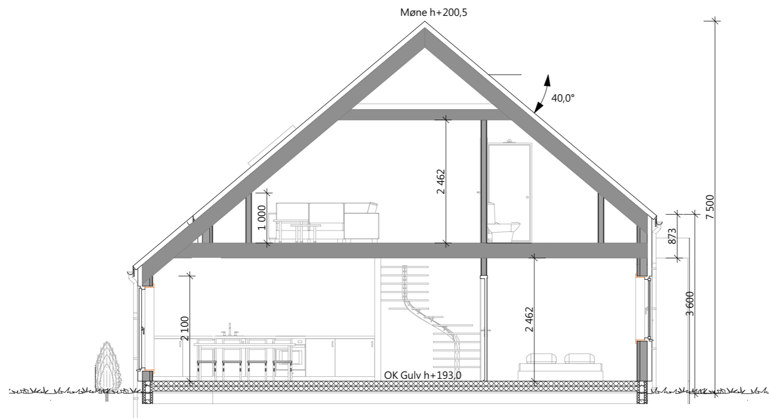
Snitt A-A
