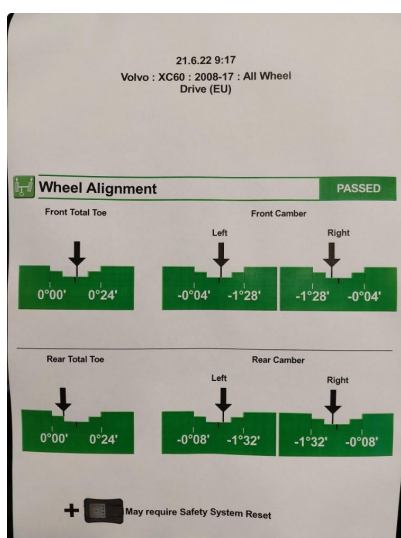
2.1 4-hjulsmåling/forstillingskontroll
