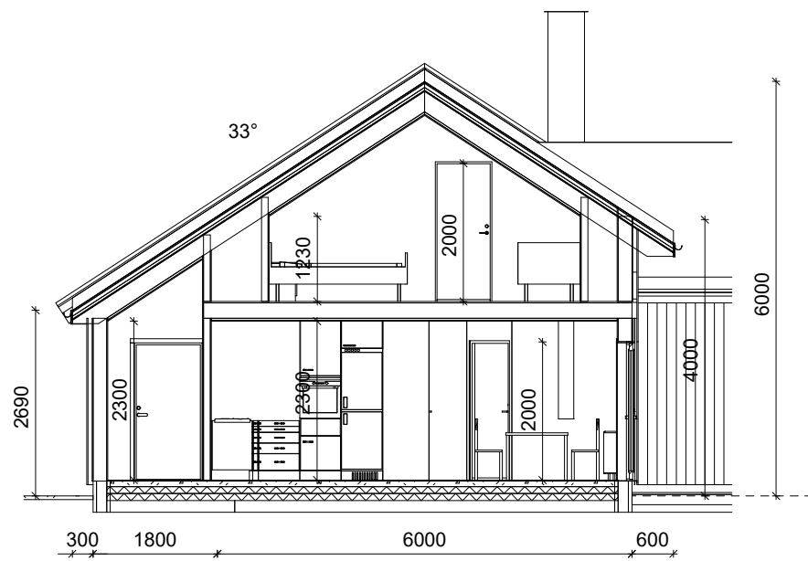
Snitt A-A
