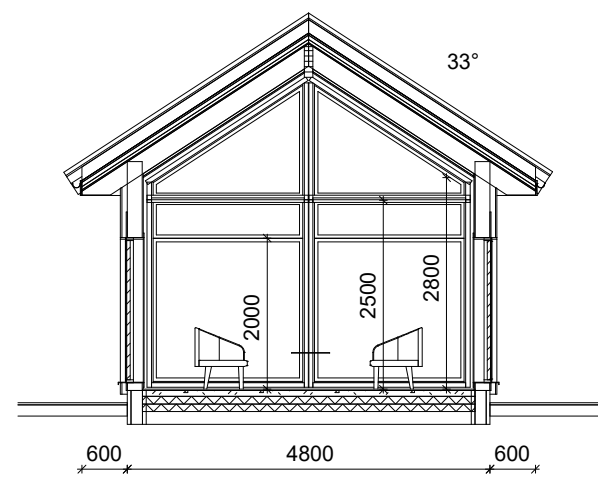
Snitt B-B
