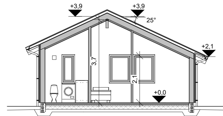
B 1 : 100
