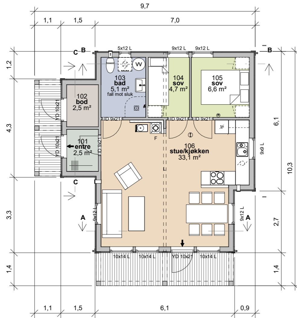
1. Etasje 1 : 100
