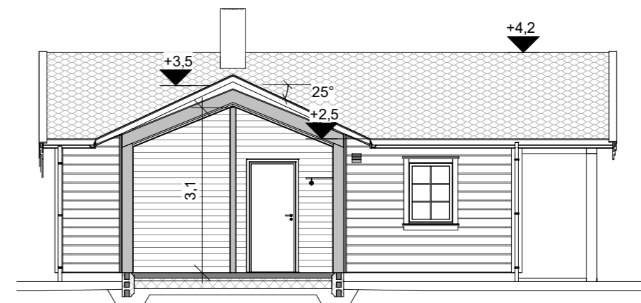
C 1 : 100
