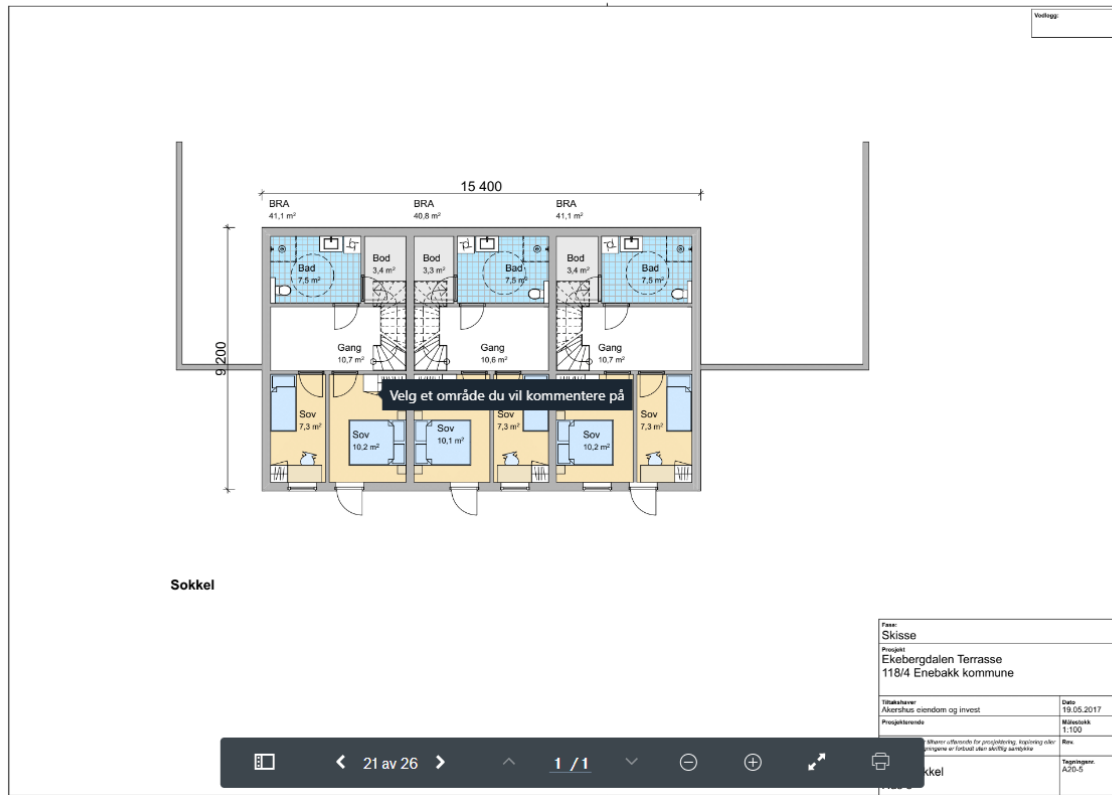
A20-5 Plan Sokkel_Hus 3.pdf
