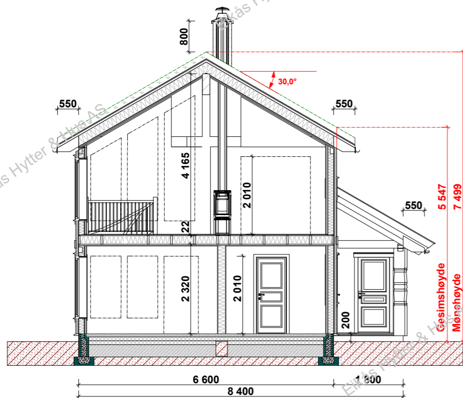
Snitt A-A
