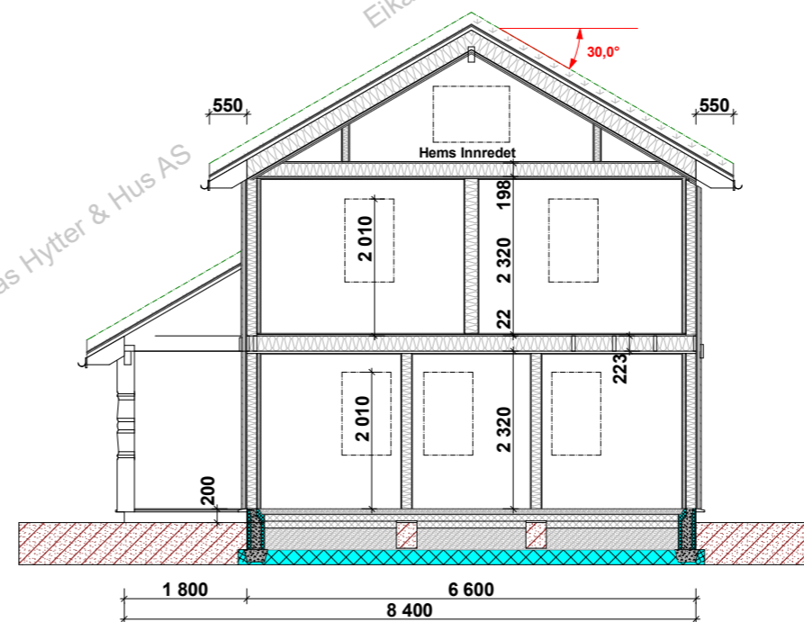
Snitt B-B
