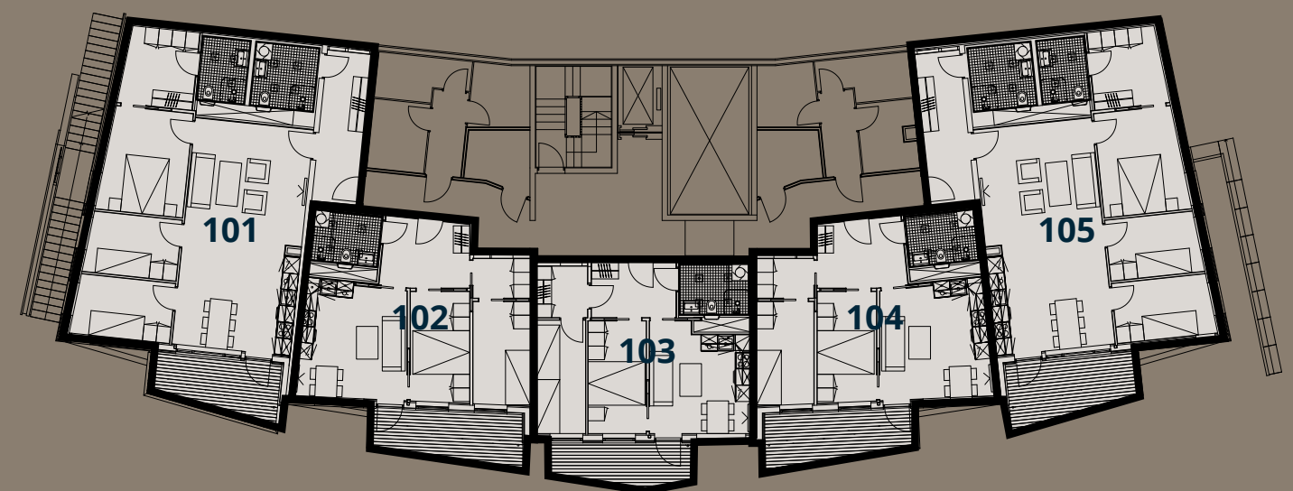
1. ETG.
