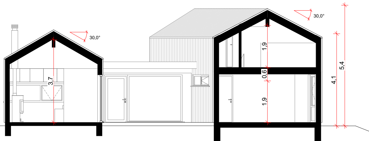
SNITT A
