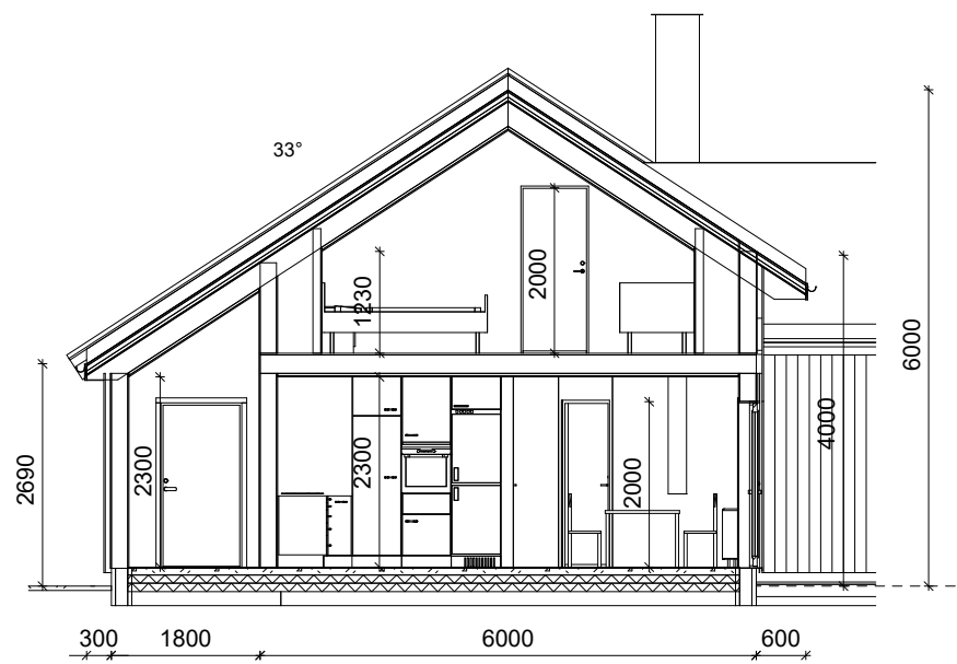
Snitt A-A
