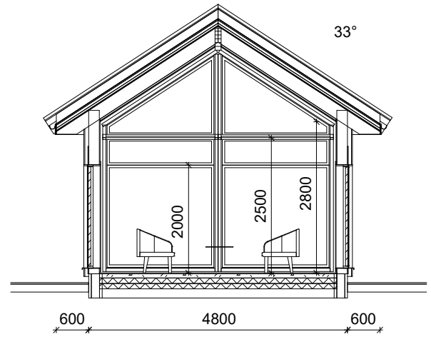
Snitt B-B
