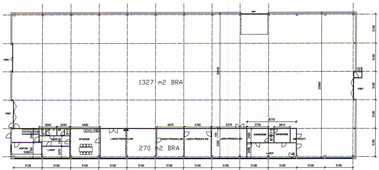
PLAN 1 Angitt bruksareal = areal innvendig vegg
