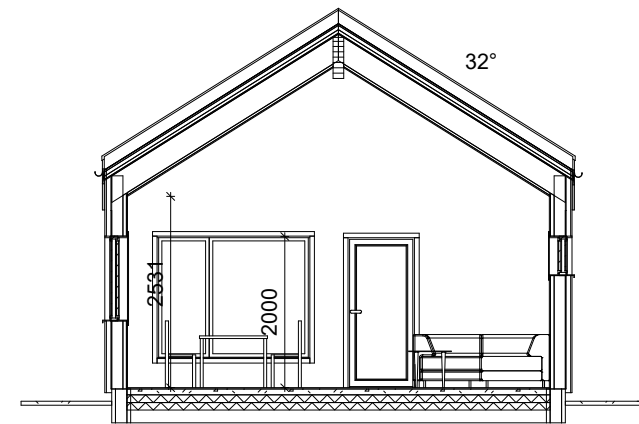
Snitt B-B
