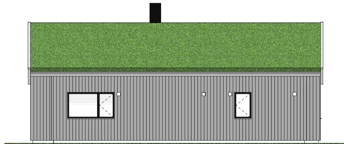
Fasade mot sør-vest
