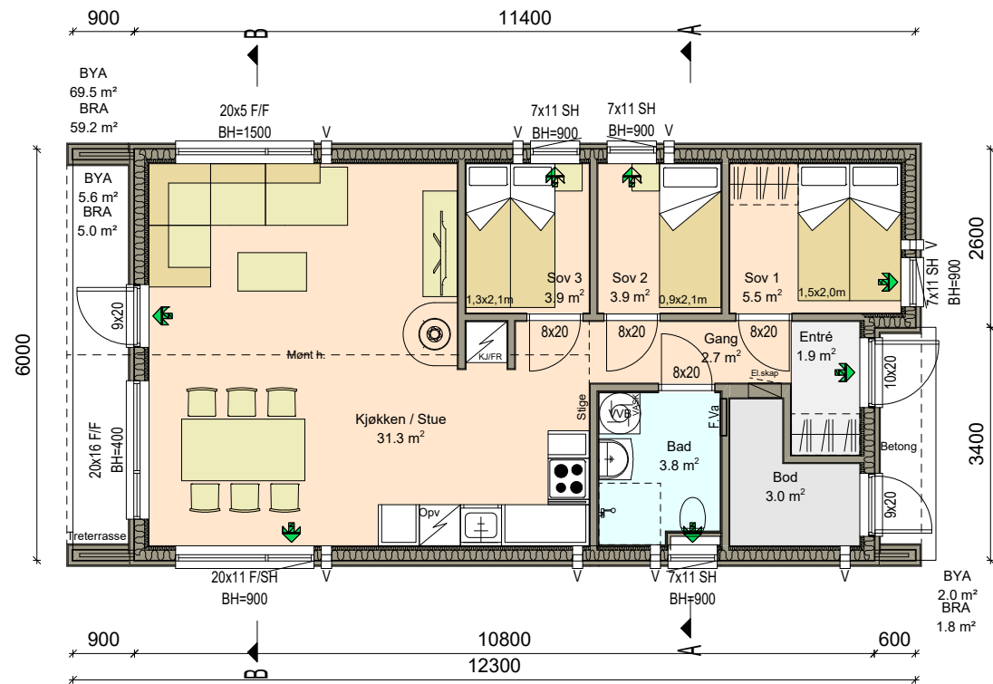
Plan 1 etg.
