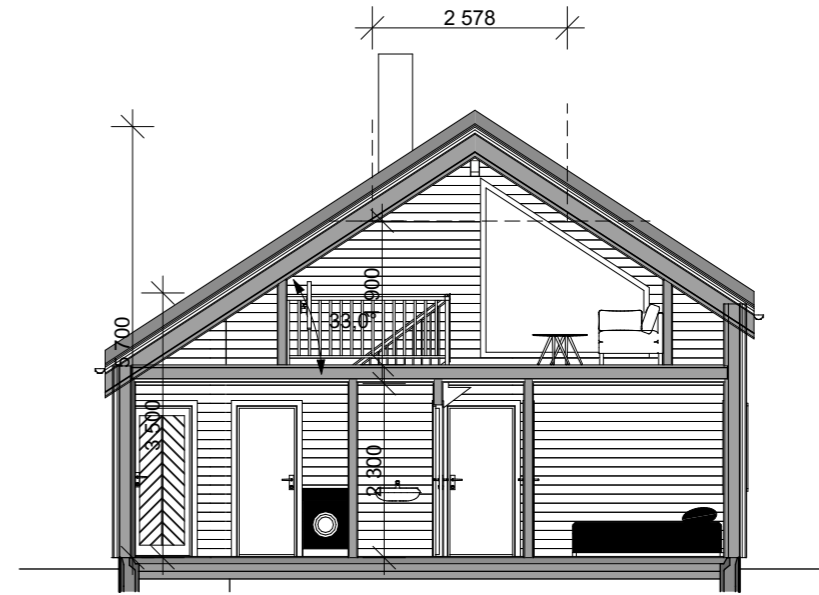
SNITT A-A
