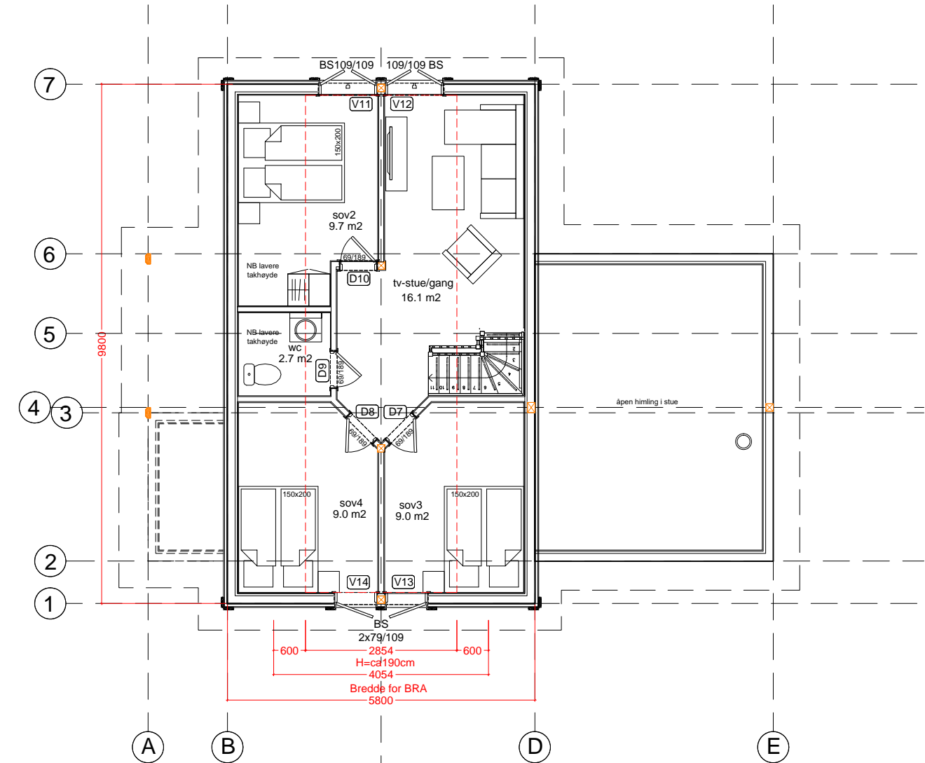
Plan 2 etg
