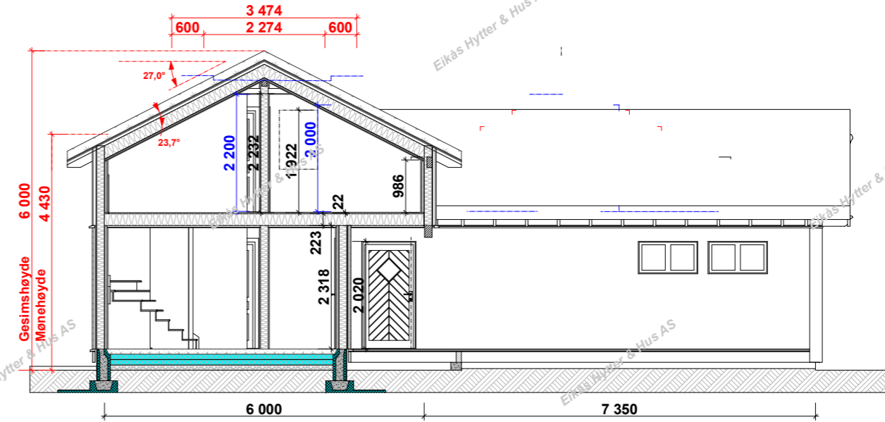
Snitt B-B
