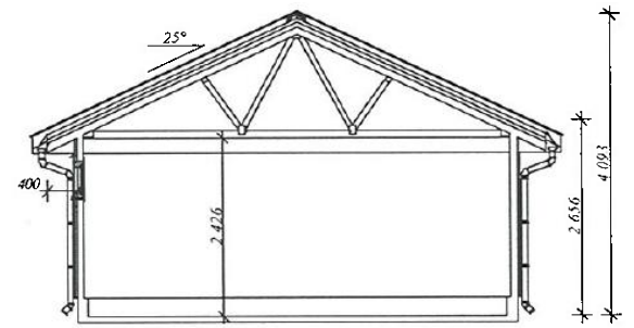
Snitt A-A
