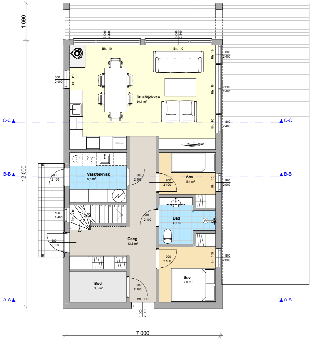
Plantegning 1. etasje
