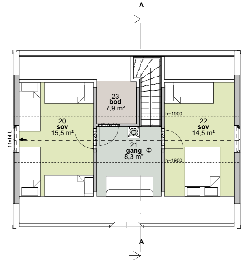
2. Etasje 1 : 100
