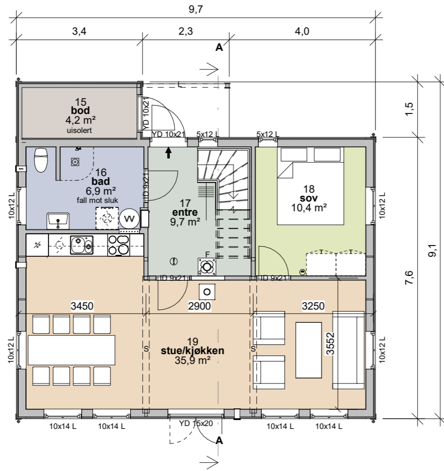
1. Etasje 1 : 100
