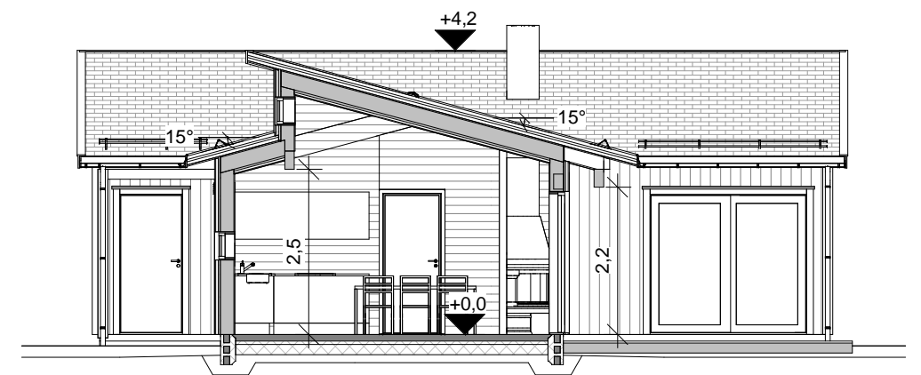
B 1 : 100
