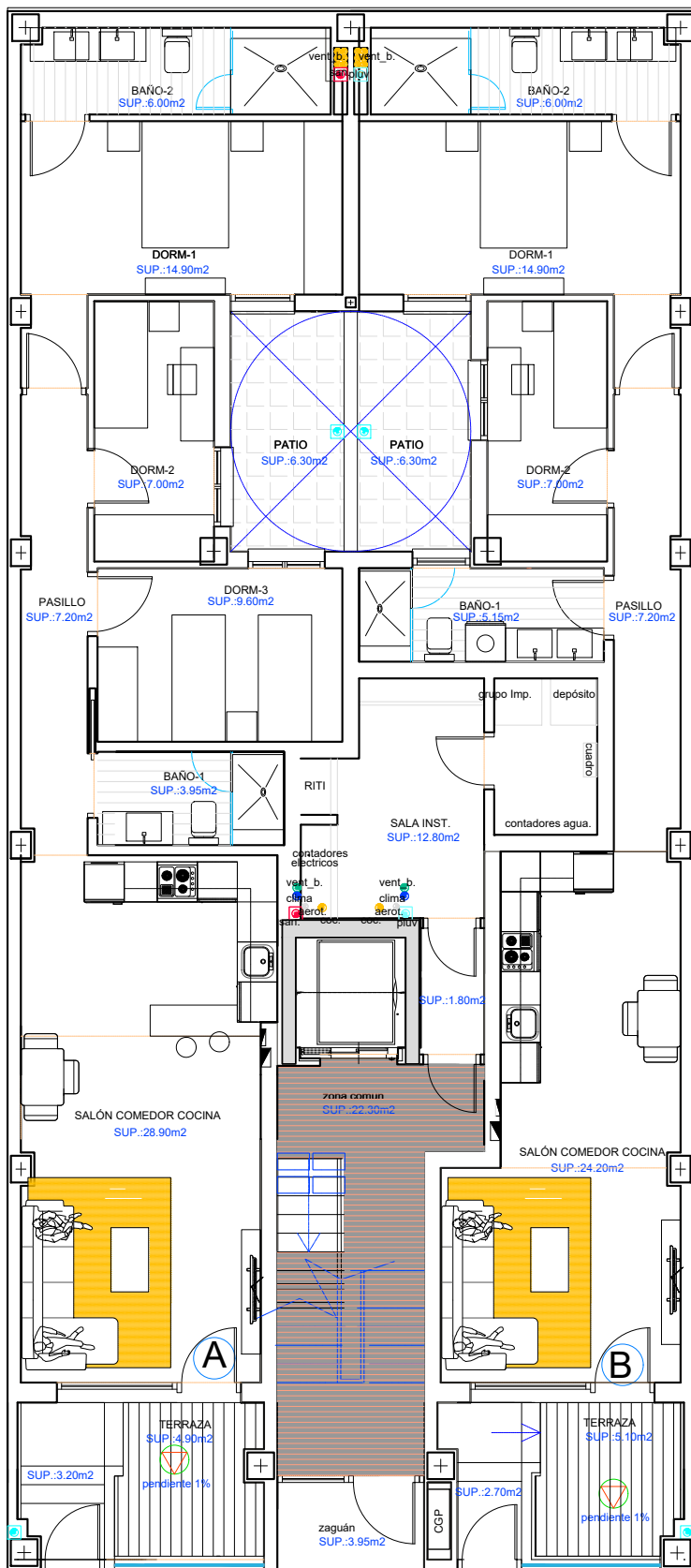
PLANTA BAJA
