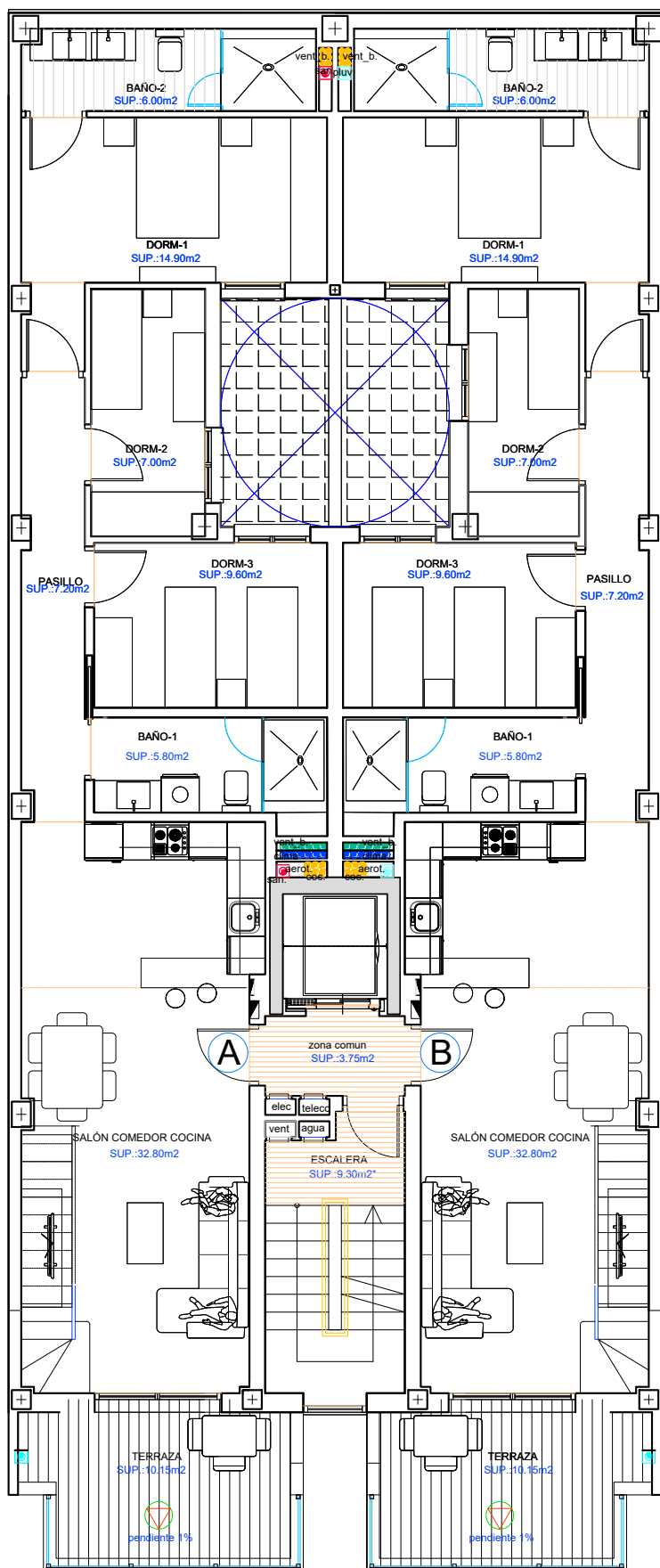
PLANTA ATICO
