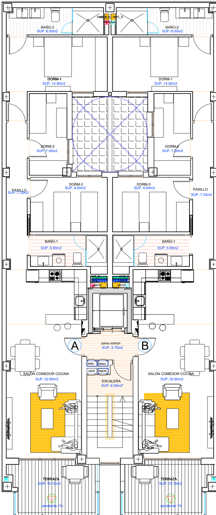
PLANTA 1-4
