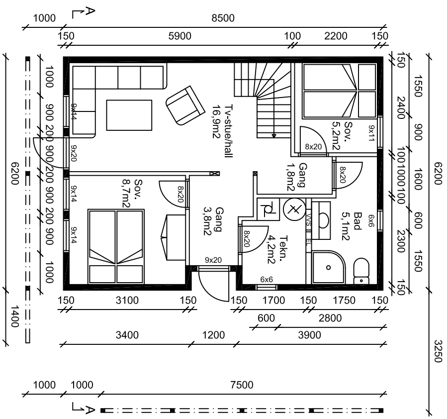
HOVEDPLAN
