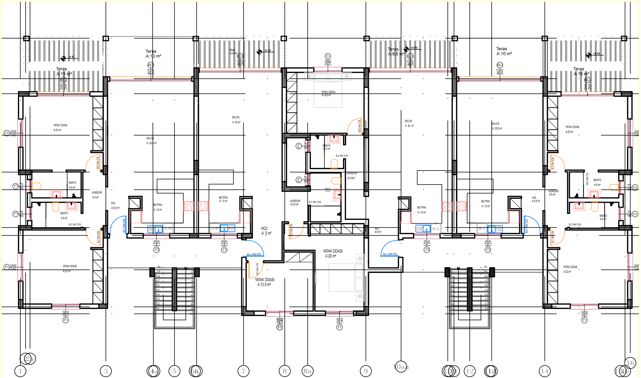
C BLOK ZEMİN KAT PLANI
