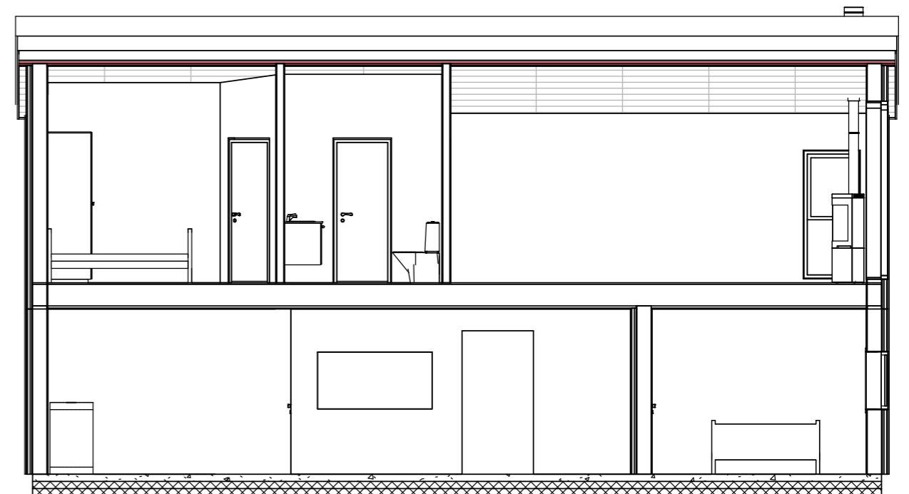
B 1 : 75
