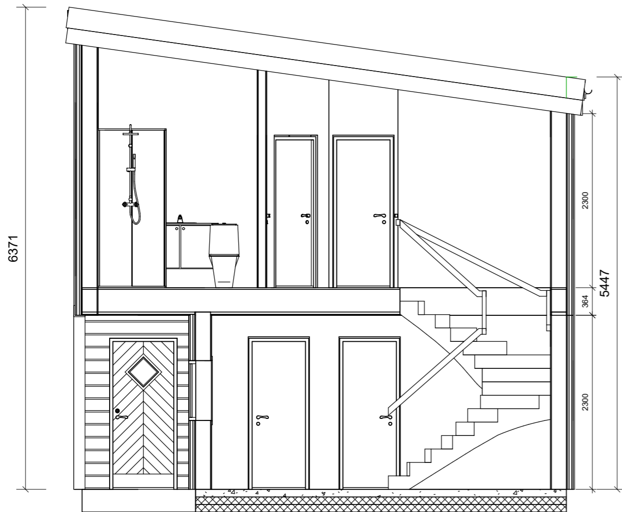
A 1 : 50
