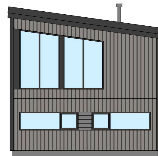
Fasade 2 1 : 100
