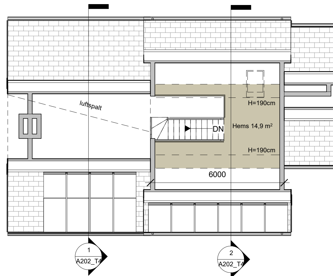
2 Hems 1 : 100
