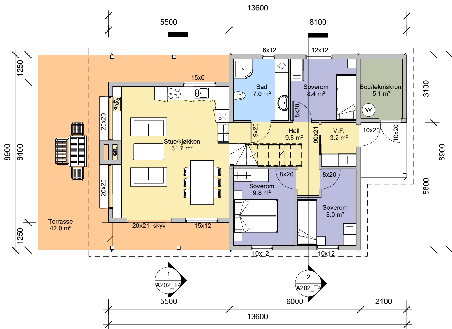
1 1 etg 1 : 100
