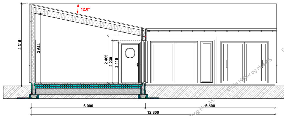
Snitt A-A
