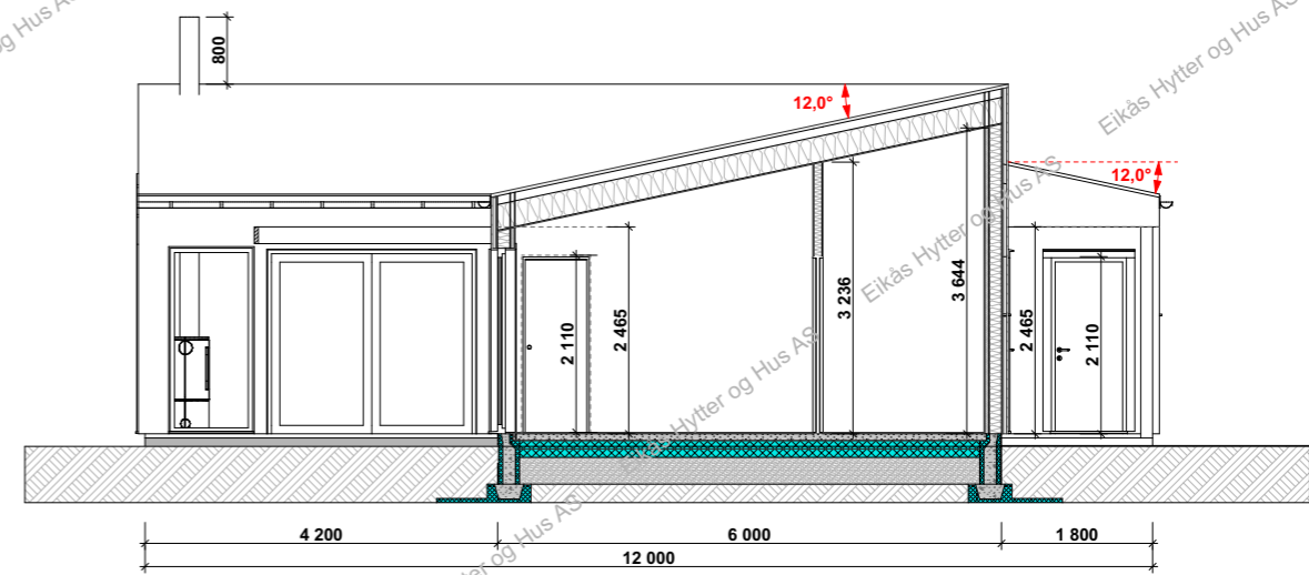
Snitt B-B
